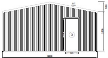
3 REAR ELEVATION 2 SCALE: 1:50 FRAME #3
